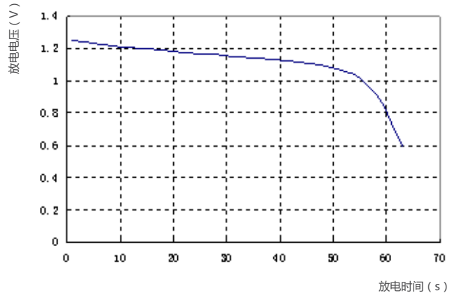
低温启动性能曲线 (-35°C)
