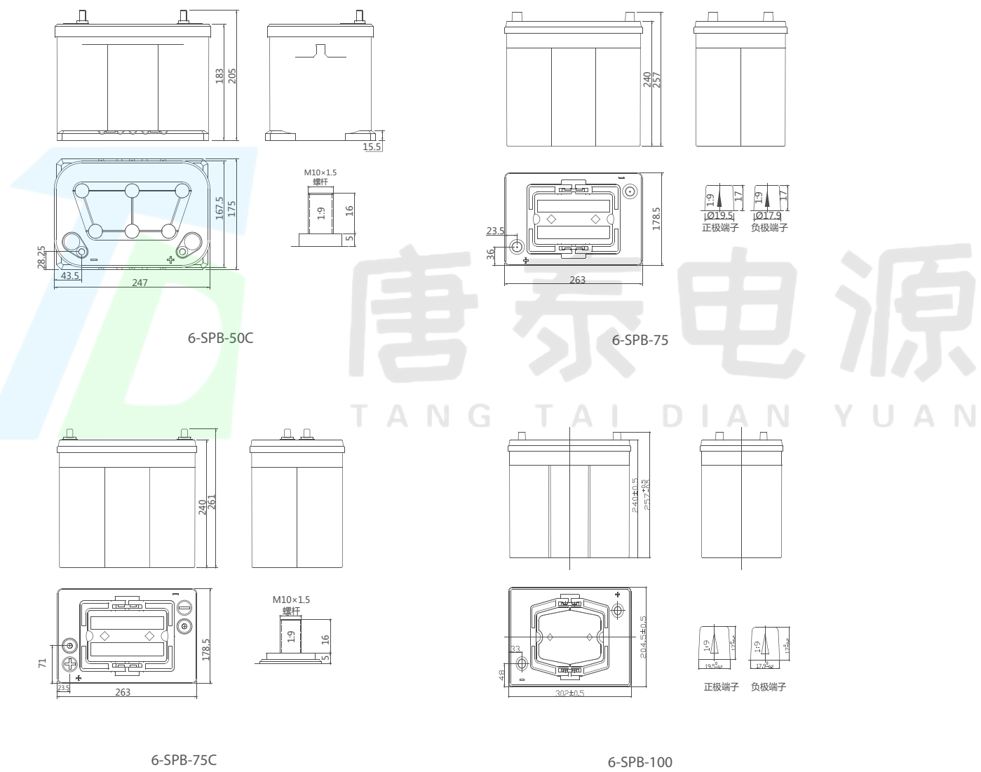
外轮廓图
