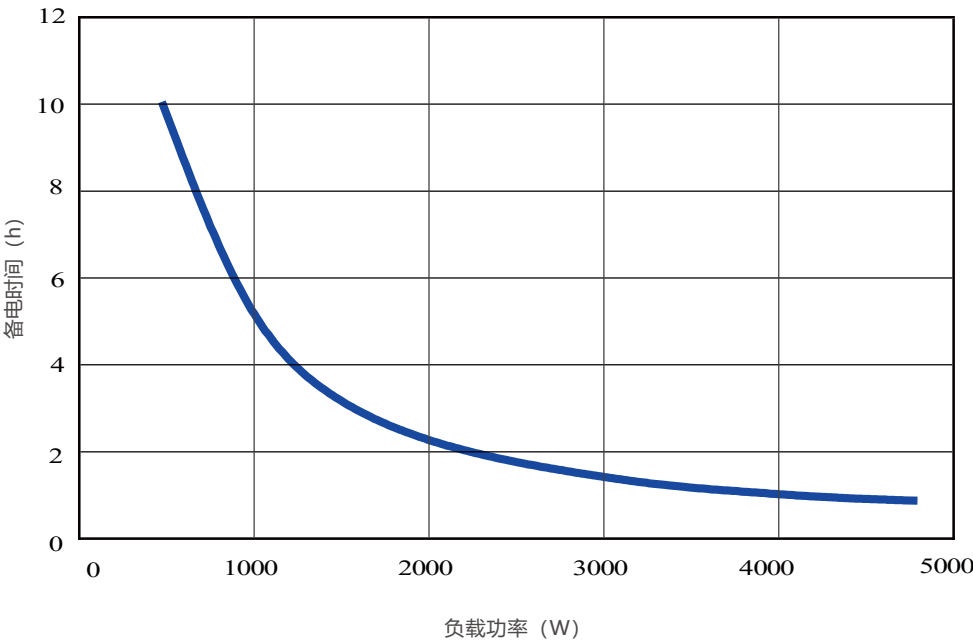
放电功率曲线
