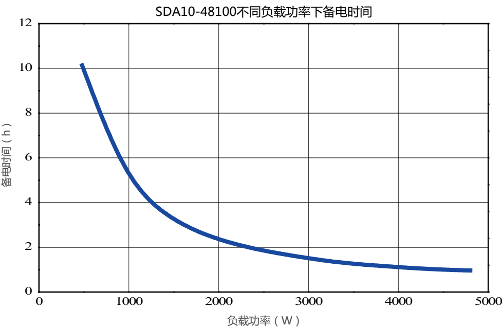
放电功率曲线
