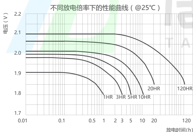
性能曲线
